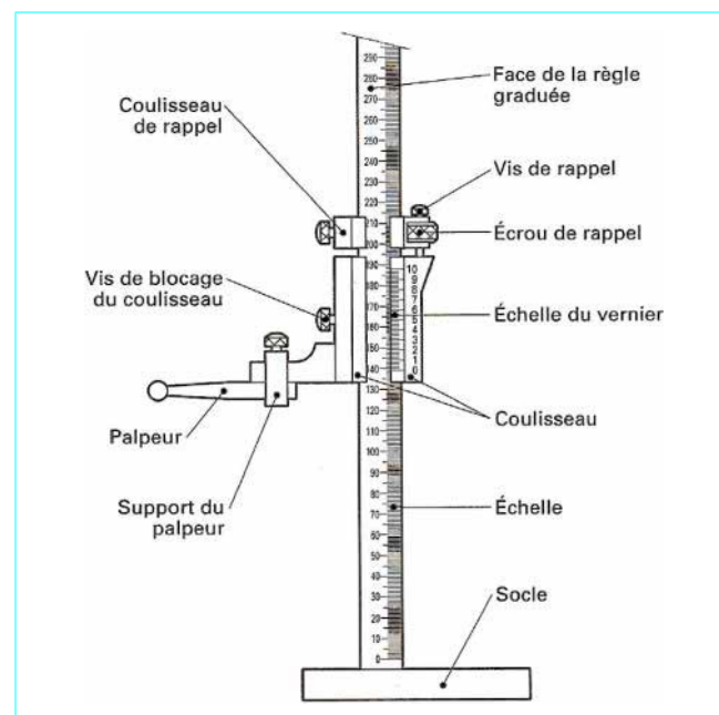
Figure 22—Trusquin de mesure à vernier
