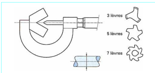
Figure 13—Micromètre à exécutions spéciales à touche fixe en vé
