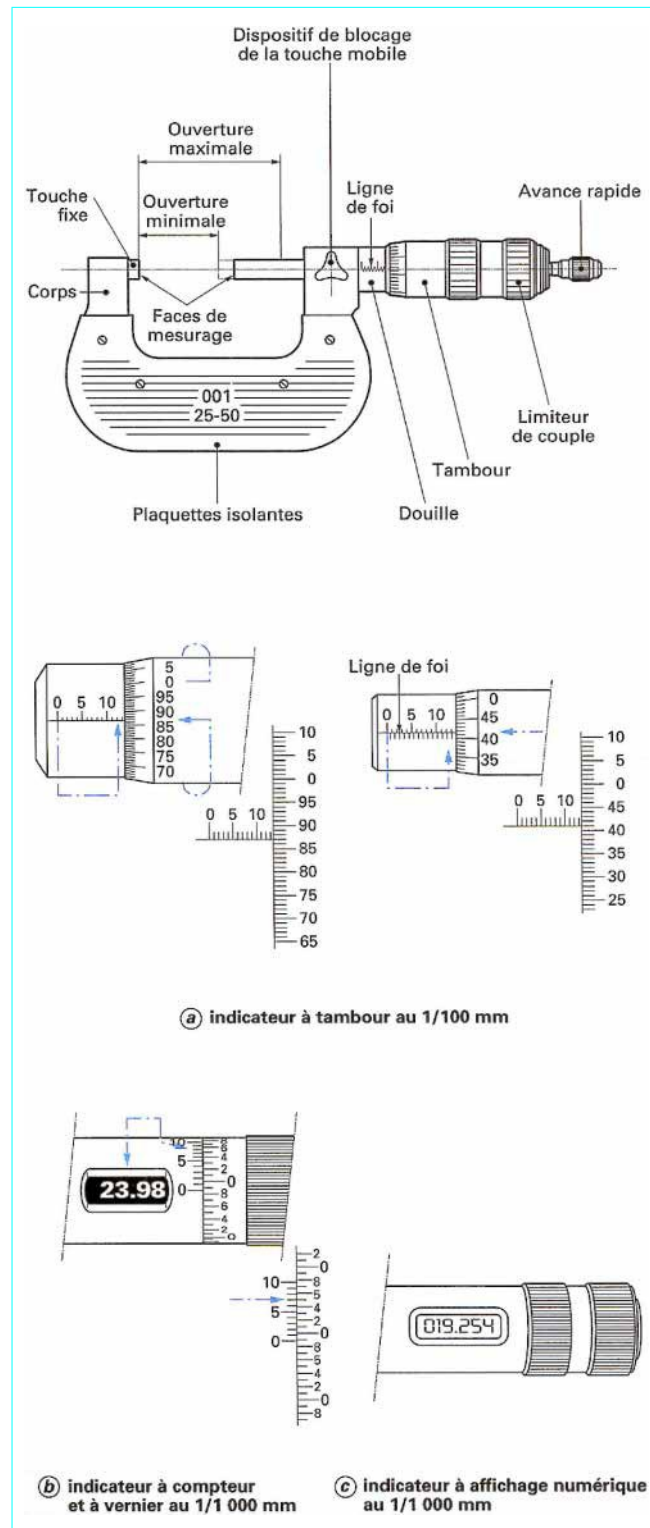
Figure 6—Schéma de principe des micromètres d'extérieur à vis
