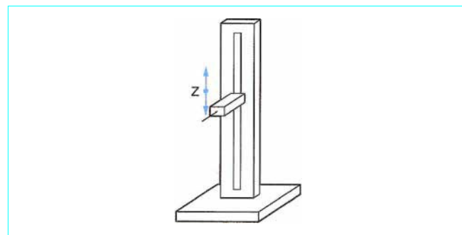
Figure 24—Schéma de principe d'une colonne de mesure verticale
