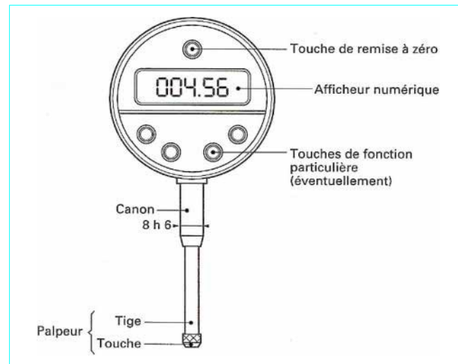
Figure 27—Schéma de principe d'un comparateur à affichage numérique
