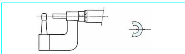
Figure 11—Micromètre à exécutions spéciales pour la mesure de parois de tubes
