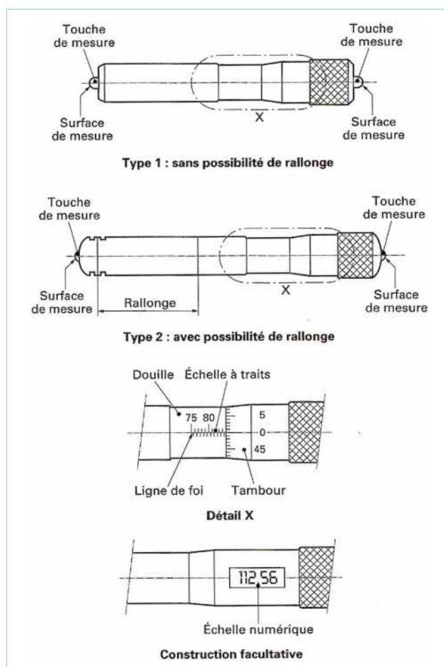
Figure 17—Schéma de principe des jauges micrométriques à deux touches
