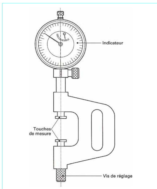
Figure 21—« C » de mesure à comparateur
