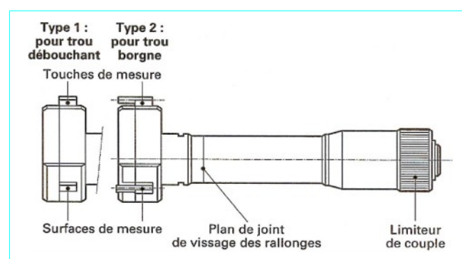
Figure 18—Schéma de principe des alésomètres (trois touches)
