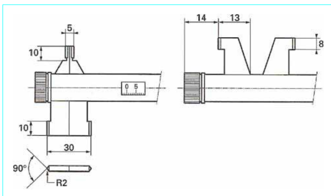
Figure 14—Micromètre d'intérieur à becs
