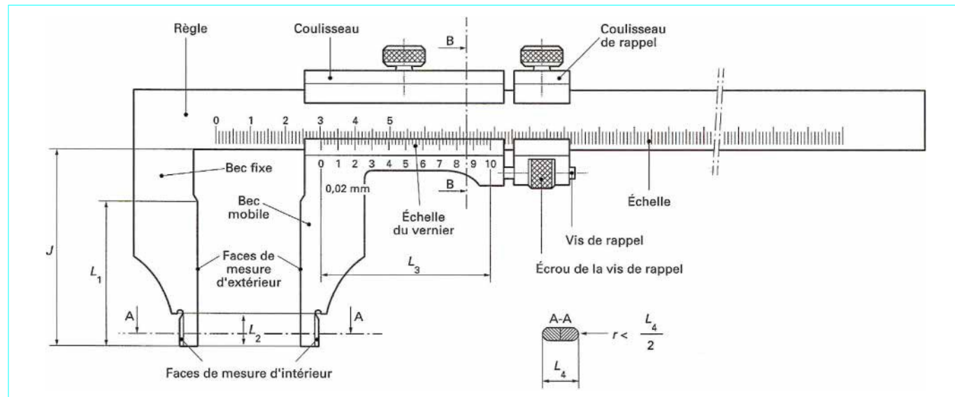
Figure 2—Pied à coulisse à vernier
