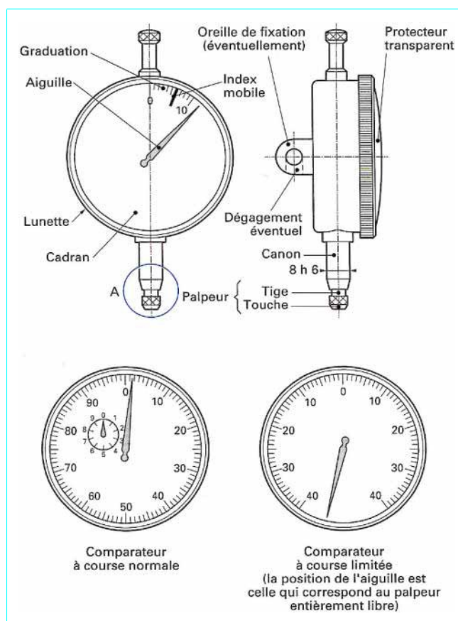
Figure 25—Schéma de principe de comparateur à tige rentrante radiale
