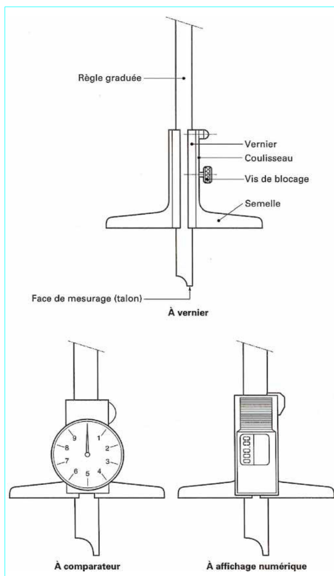
Figure 5—Schéma de principe des jauges de profondeur à coulisse
