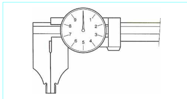
Figure 3—Pied à coulisse à comparateur
