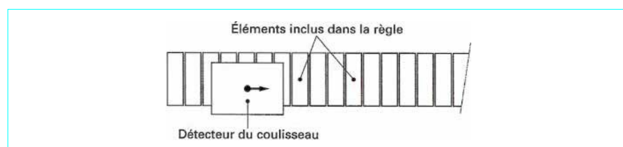
Figure A—Principe d'une règle capacitive
