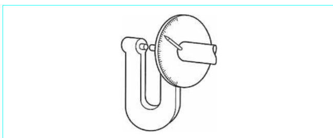
Figure 10—Micromètre à exécutions spéciales de lamineur
