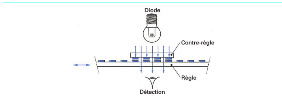
Figure B—Principe d'une règle incrémentale
