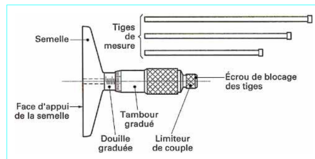
Figure 16—Schéma de principe d'une jauge de profondeur à vis
