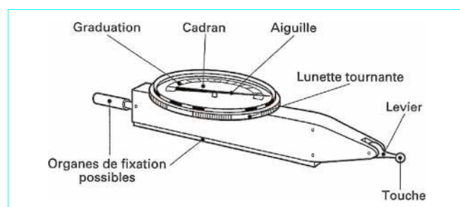
Figure 26—Schéma de principe d'un comparateur à levier
