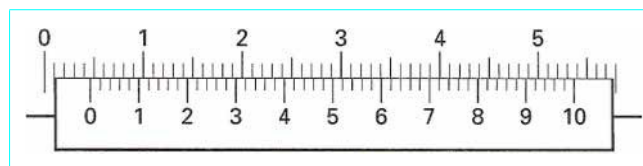
Figure 1—Exemple de vernier au 1/50 mm
