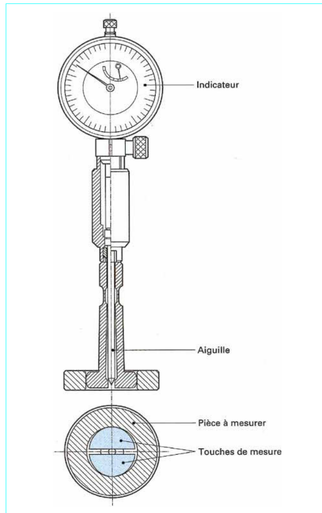
Figure 20—Mesureur d'alésage à aiguille
