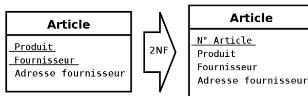
Figure 2.35- Exemple de normalisation en deuxième forme normale. On suppose qu'un même fournisseur peut fournir plusieurs produits et qu'un même produit peut être fourni par différents fournisseurs.
