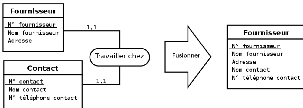
Figure 2.29 - Lorsque les cardinalités d'un type association sont toutes 1, 1 c'est qu'il s'agit d'un type association fantôme.
