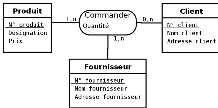
Figure 2.16 - Le type-association Commande lie les type-entités Produit , Client et Fournisseur .
