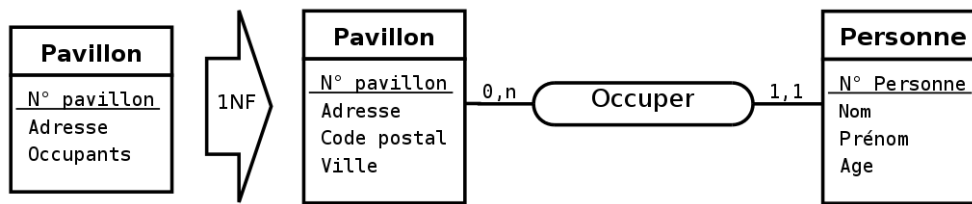
Figure 2.34- Exemple de normalisation en première forme normale.
