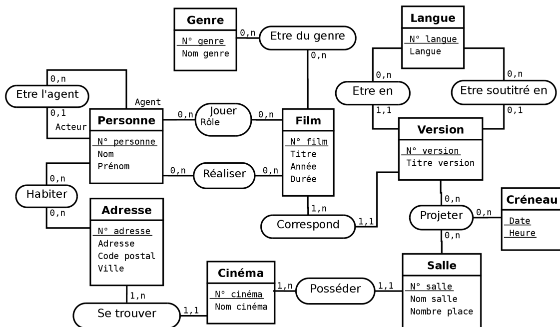
Exemple de MCD répondant à la question 2.7.1 du TD 2.7
