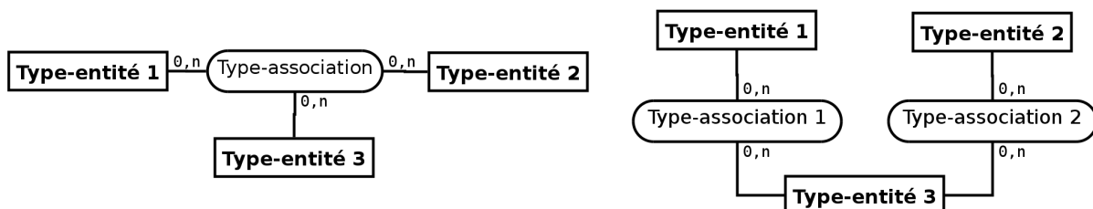
Figure 2.18 - Ces deux modélisations ne sont pas des alternatives.
