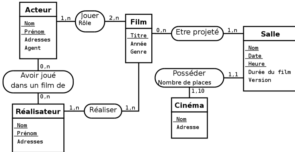
Figure 2.38 – Ce modèle entités/associations n'est pas en bonne forme!
