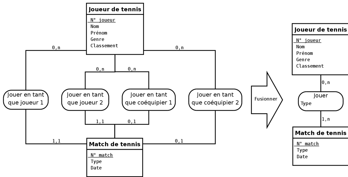
Figure 2.28 - Un seul type association suffit pour remplacer les quatre type associations Jouer en tant que ...
