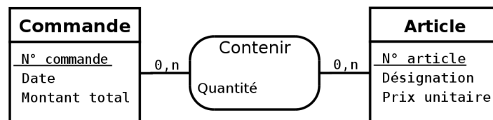
Figure 2.23 - Il faut supprimer l'attribut Montant total du type-entité Commande car on peut le calculer à partir des attributs Quantité du type association Contenir et Prix unitaire du type-entité Article.
