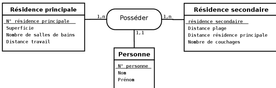
Figure 2.17 - Modélisation des résidences principales et secondaires d'un ensemble de personnes.
