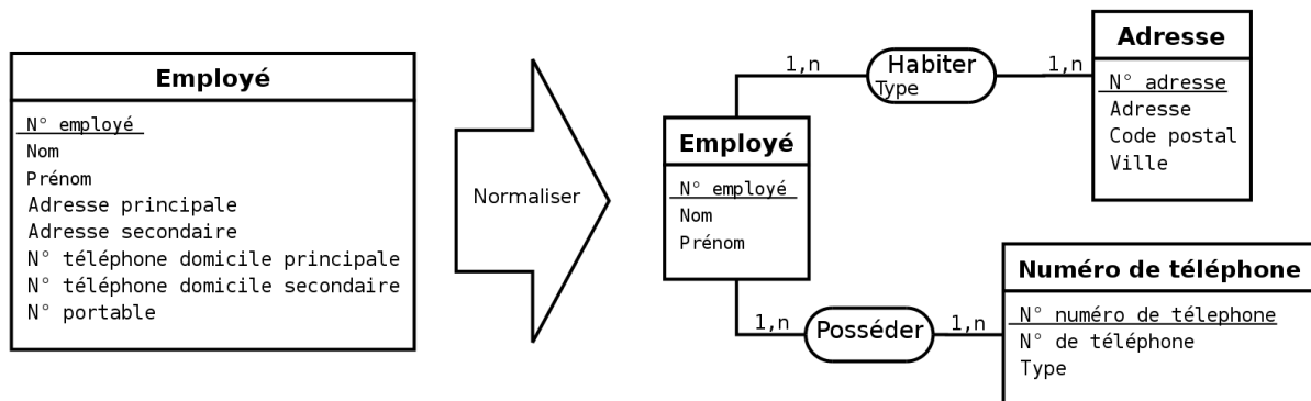
Figure 2.22 - Remplacement des attributs multiples en un type-association et un type-entité et décomposition des attributs composites.
